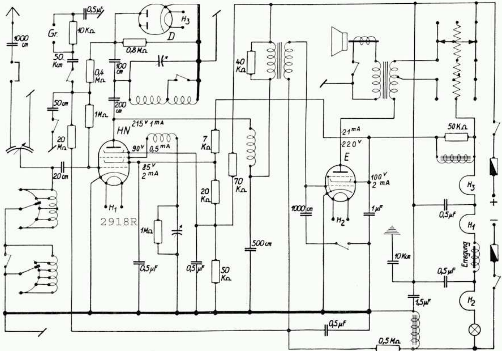
Lumophon, Markgraf G, Gleichstrom, 1 Kreis
